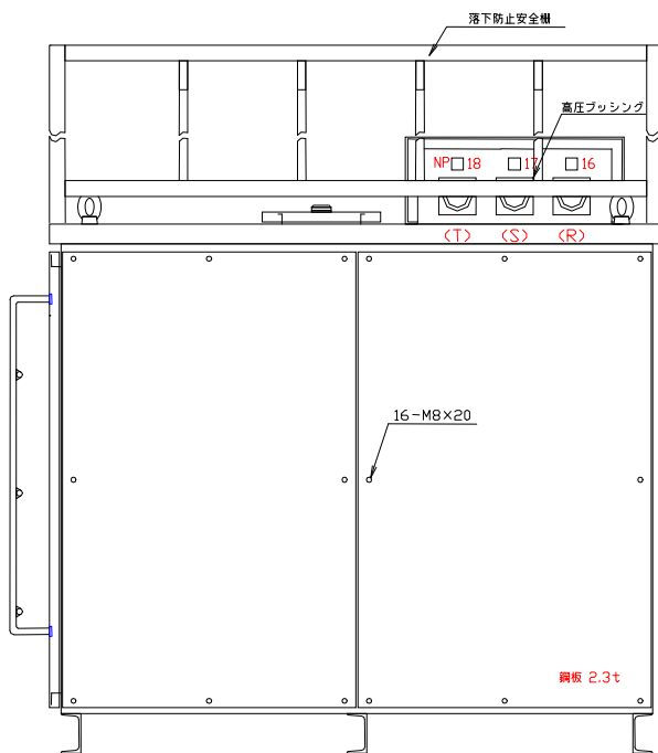
背面図 1555
