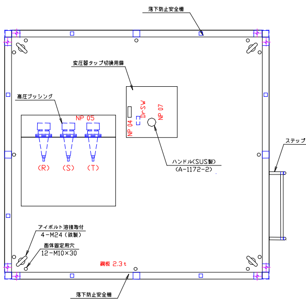
正面
