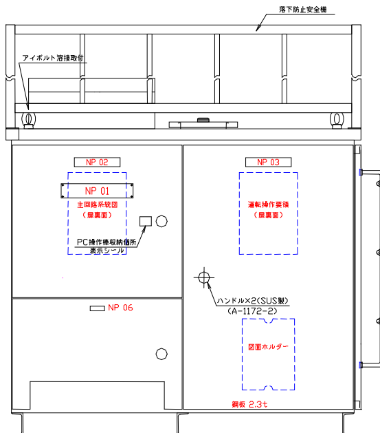
正面図
